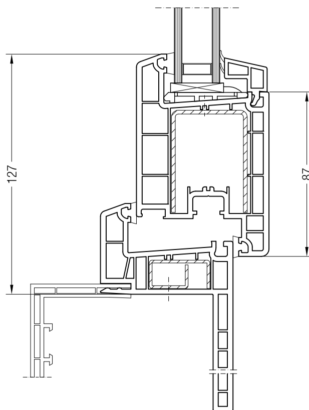
Коробка для санации 40 или 60, 550570 или 550550 и створка Z 87, 550760
