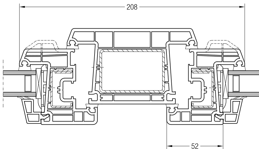
Импост 120, 550780 и створка Z 52, 550480 или створка A 52, 550040
