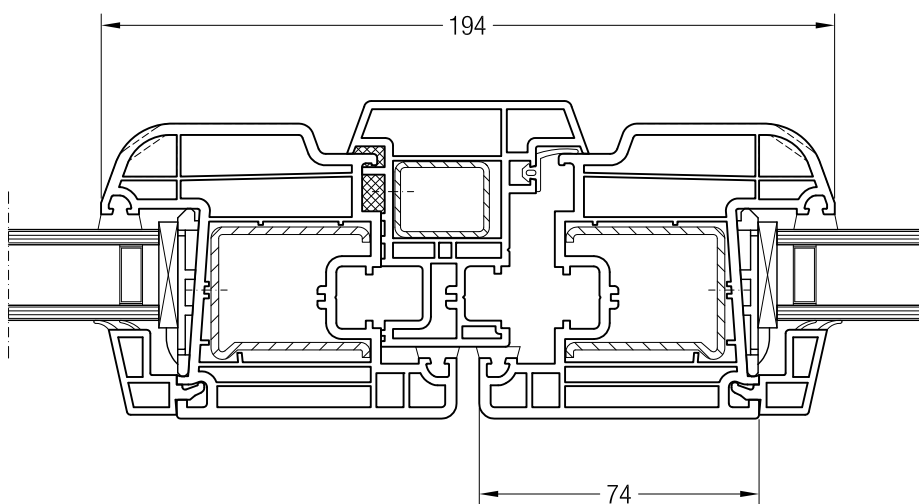
Ложный импост №1, 550535 и створка A 74, 550390 или створка 74 круглая, 550070
