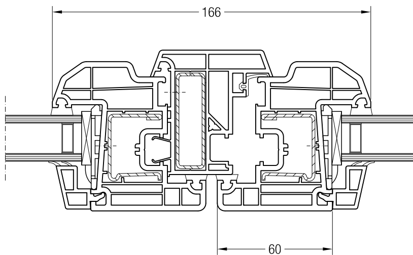
Ложный импост 70, 550775 и створка A 60, 550050
