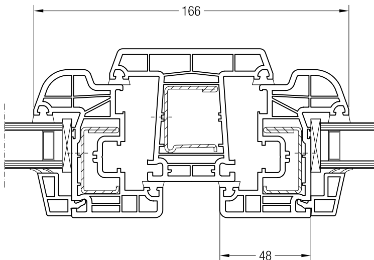
Импост 86, 550020 и створка 48 круглая, 550481
