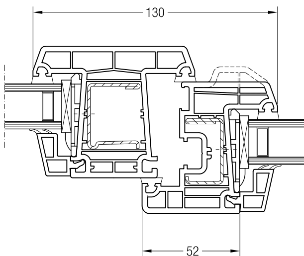
Импост 86, 550020 и створка Z 52, 550480 или створка A 52, 550040
