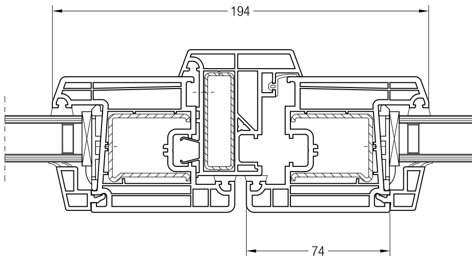
Ложный импост 70, 550775 и створка Z 74, 550510
