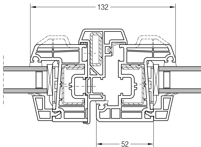
Штульп 70, 550085 и створка Z 52, 550480 или створка A 52, 550040
