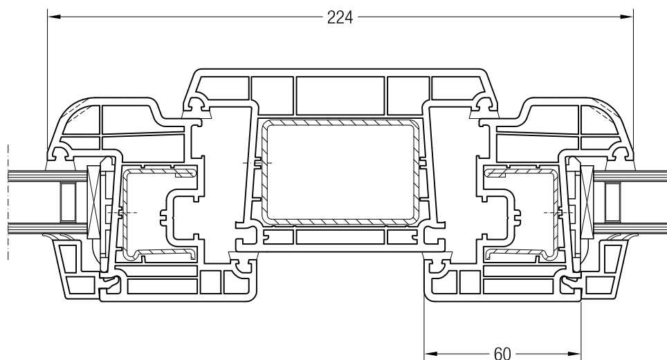
Импост 120, 550780 и створка A 60, 550050 или створка 60 круглая, 550060
