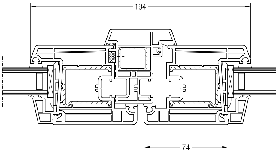
Ложный импост №1, 550535 и створка Z 74, 550510
