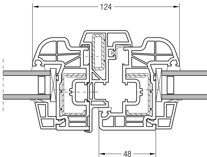
Штульп 70, 550085 и створка 48 круглая, 550481
