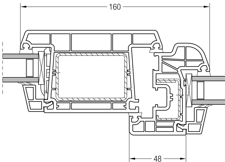
Импост 120, 550780 и створка 48 круглая, 550481
