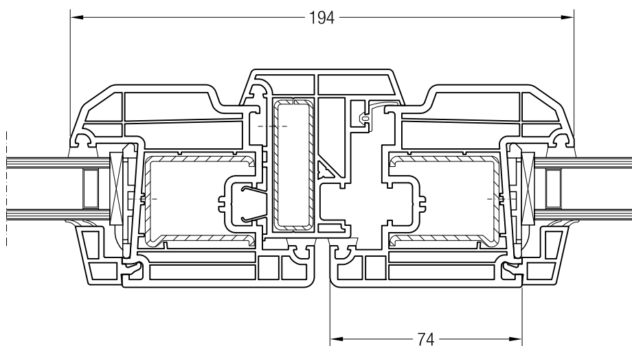
Ложный импост 70, 550775 и створка A 74, 550390
