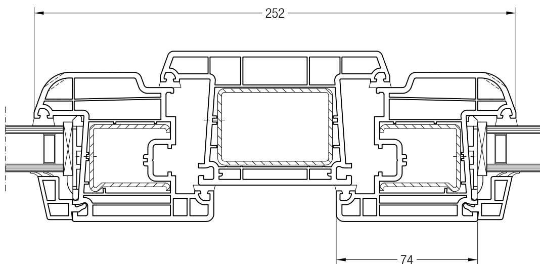
Импост 120, 550780 и створка А 74, 550390 или створка 74 круглая, 550070
