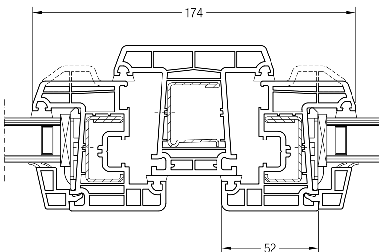
Импост 86, 550020 и створка Z 52, 550480 или створка A 52, 550040
