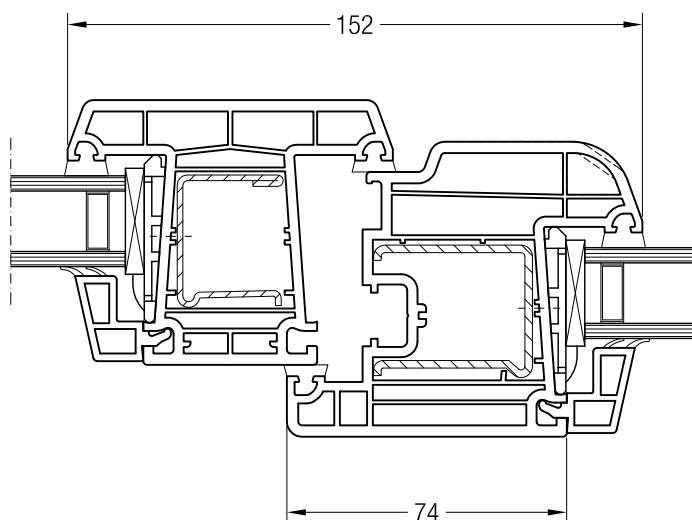
Импост 86, 550020 и створка A 74, 550390 или створка 74 круглая, 550070
