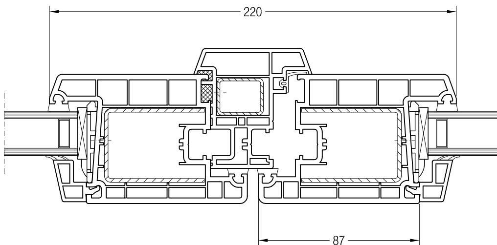
Ложный импост №1, 550535 и створка Z 87, 550760
