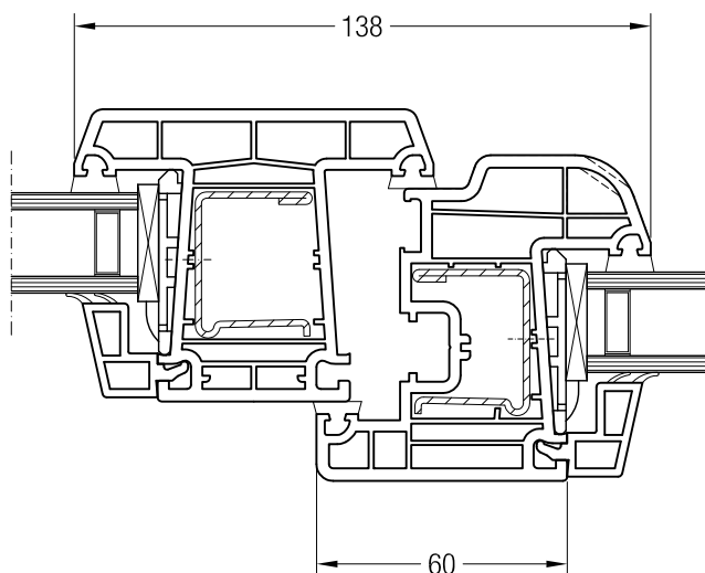
Импост 86, 550020 и створка A 60, 550050 или створка 60 круглая, 550060
