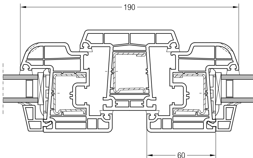
Импост 86, 550020 и створка A 60, 550050 или створка 60 круглая, 550060
