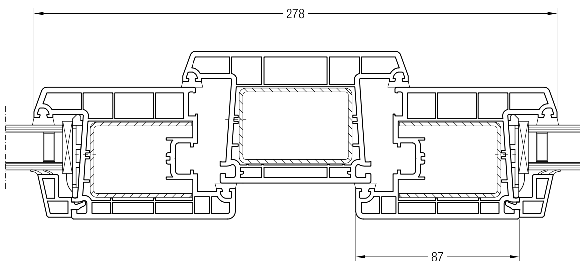
Импост 120, 550780 и створка Z 87, 550760
