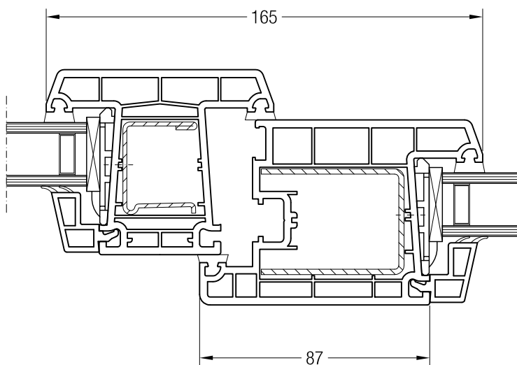
Импост 86, 550020 и створка Z 87, 550760
