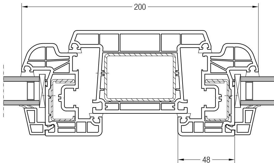
Импост 120, 550780 и створка 48 круглая, 550481
