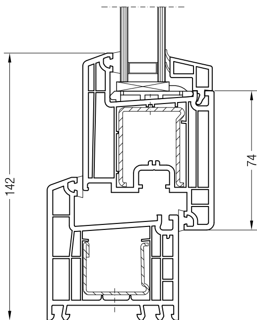
Коробка 76-2, 550680 и створка Z 74, 550510
