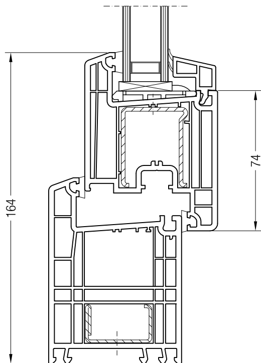
Коробка 98, 550540 и створка Z 74, 550510
