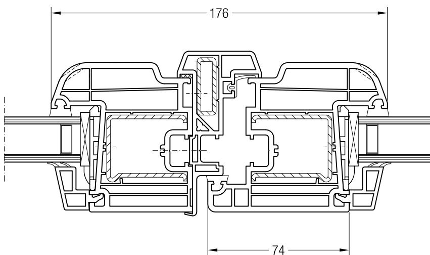
Штульп 70, 550085 и створка A 74, 550390 или створка 74 круглая, 550070
