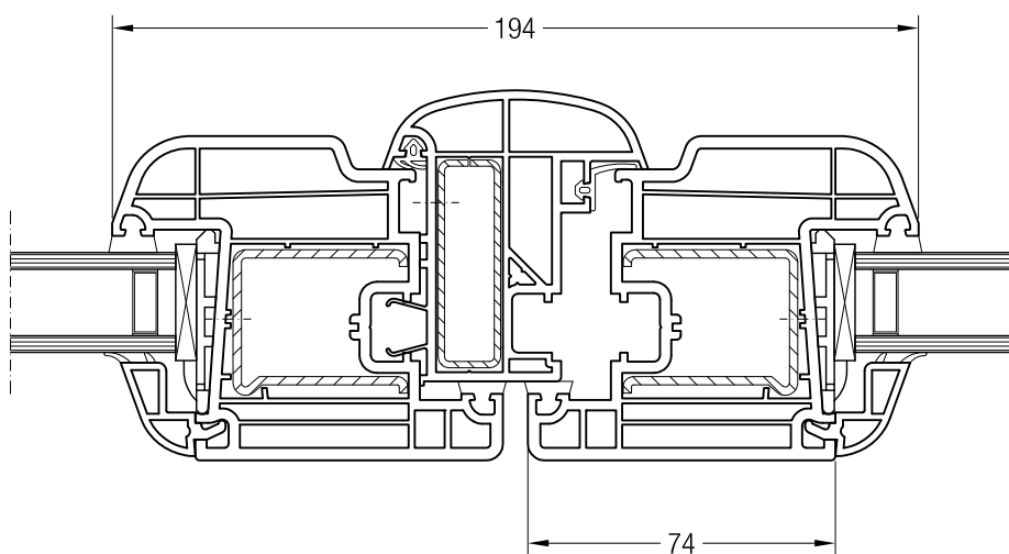
Ложный импост 70 круглый, 550536 и створка 48 круглая, 550481
