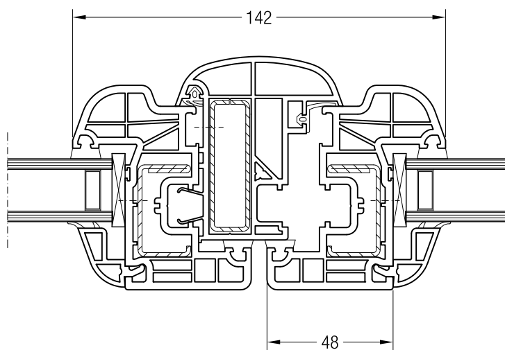
Ложный импост 70 круглый, 550536 и створка 48 круглая, 550481
