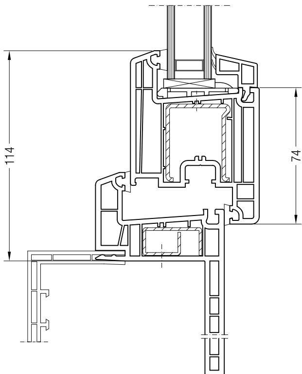
Коробка для санации 40 или 60, 550570 или 550550 и створка Z 74, 550510
