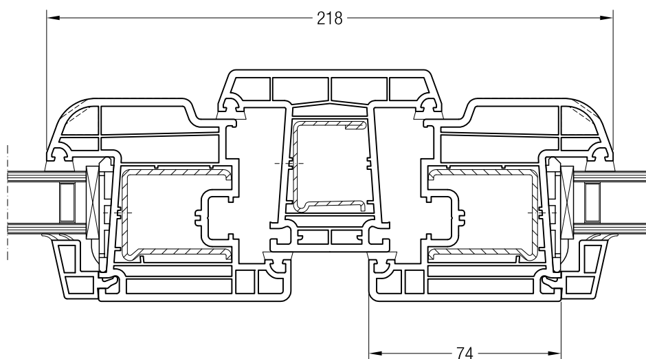
Импост 86, 550020 и створка A 74, 550390 или створка 74 круглая, 550070
