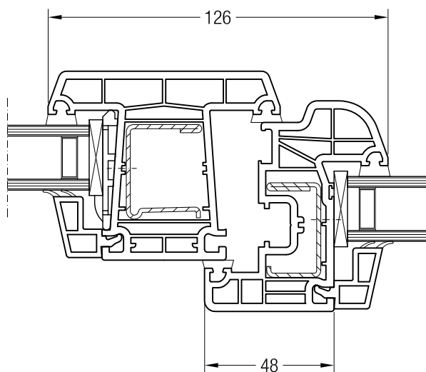
Импост 86, 550020 и створка 48 круглая, 550481
