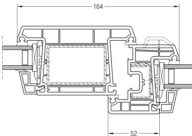
Импост 120, 550780 и створка Z 52, 550480 или створка A 52, 550040
