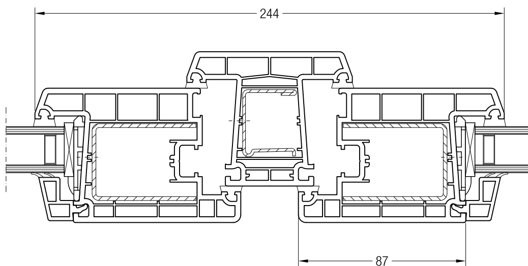
Импост 86, 550020 и створка Z 87, 550760
